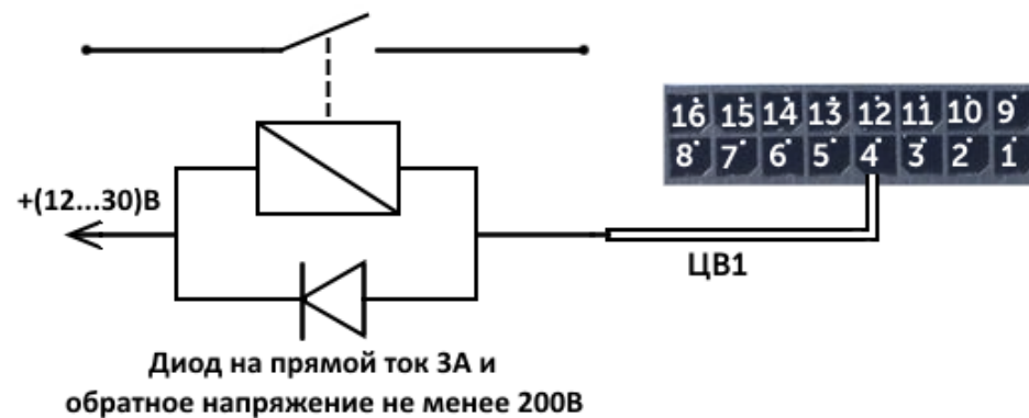
Рис. 4.6. Схема подключения реле на Цифровой выход 1.
